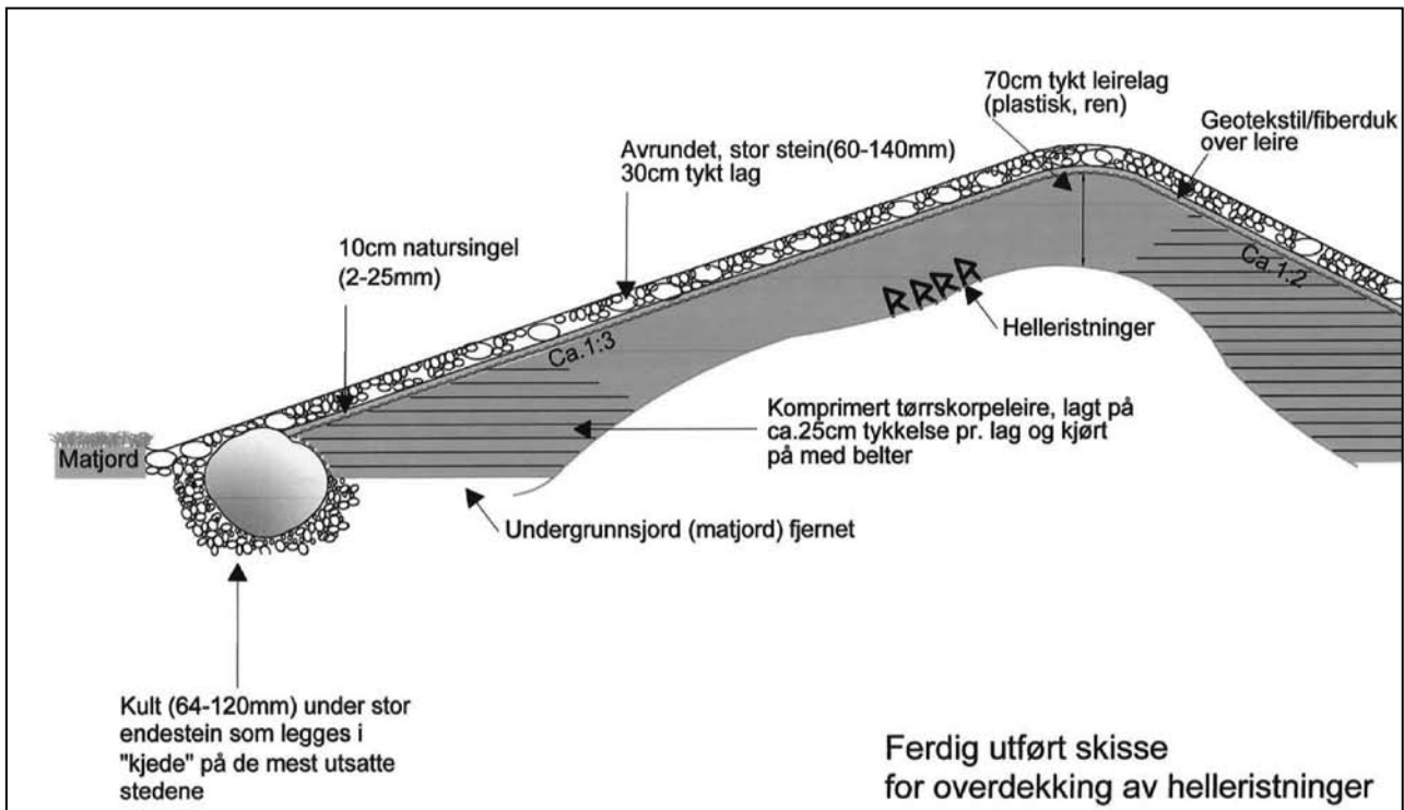
Figur 3_21: Prinsippskissa viser korleis overdekkinga vart gjennomført i praksis. Illustrasjon: Kristin Marie Berg.
