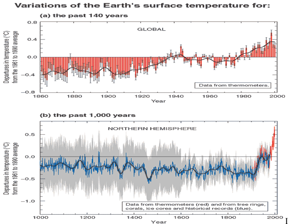
Figur 1. Endringer i temperatur basert på historiske observasjoner. Kilde: IPCC (2001).
