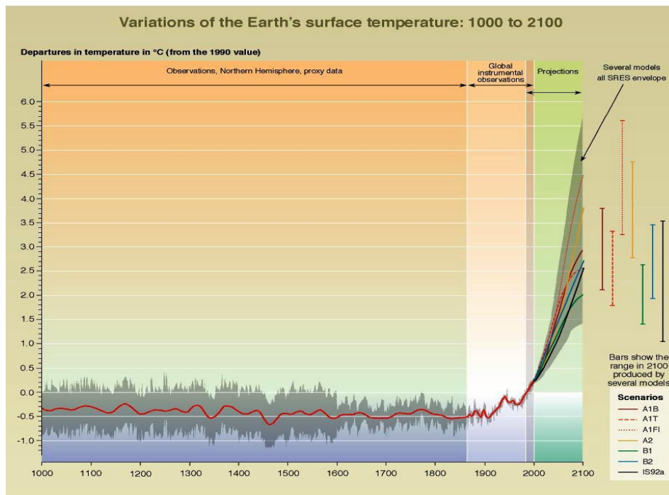
Figur 2. Observert variasjoner i global temperatur siste 1000 år samt beregninger av fremtidig oppvarming neste 100 år basert på ulike "Business as Usual"-scenarier og ulike klimamodeller. Kilde IPCC (2001).
