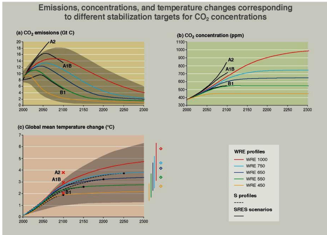
Figur 4. Utslipp, konsentrasjoner og temperaturendringer. Kilde IPCC(2001)
