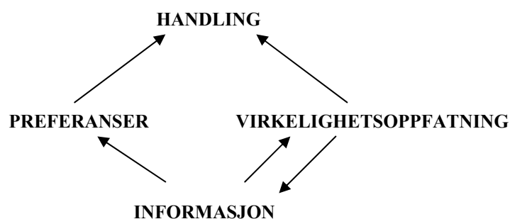
Figur 3.2 Tykk rasjonalitetsmodell
