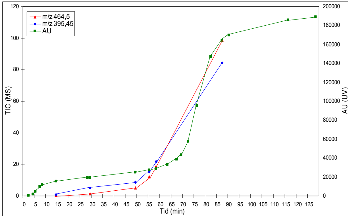
Figur 4.9: Kapasitetskurve for 2,5mg/ml HSA løst i 150mM \text{NH}_4\text{Ac} (■), med prosentvis gjennombrudd av HSA detektert på LC-MS ( m/z 464,5 og m/z 395,45).
