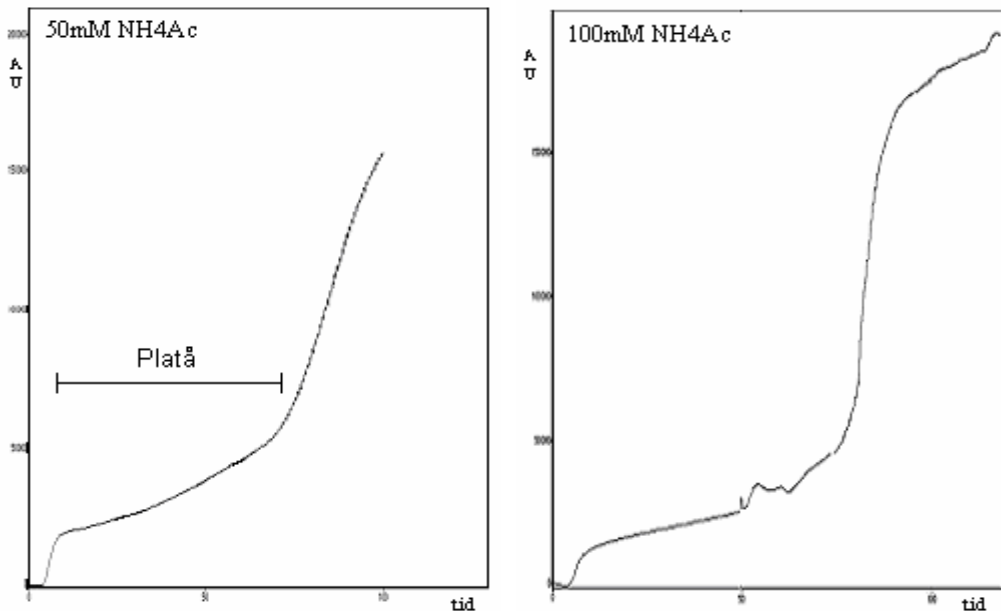
Figur 4.6: Bindingskapasitetskurve for 2,5mg/ml HSA i 50mM NH 4 Ac (venstre) og 100mM NH 4 Ac* (høyre). *Kurven er satt sammen av to kromatogram på grunn av at pumpe måtte skiftes midt i opparbeidelsen.
